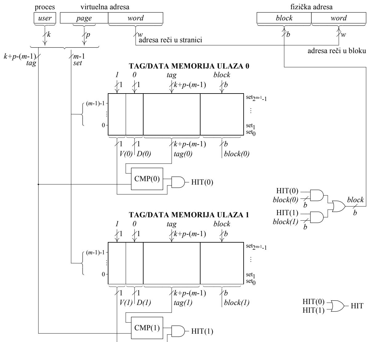
Virtuelna memorija stranične organizacije i jedinica sa set-asocijativnim preslikavanjem
