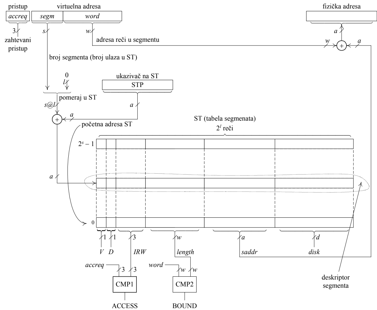
Virtuelna memorija segmentne organizacije
