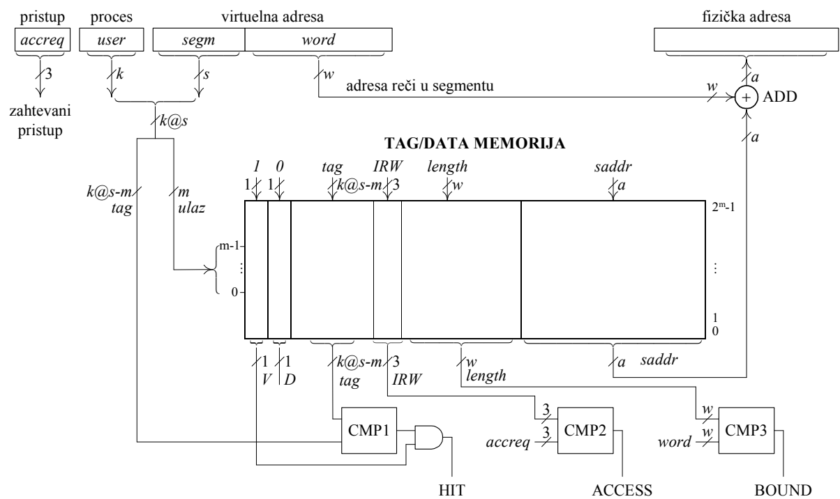
Virtuelna memorija segmentne organizacije i jedinica sa direktnim preslikavanjem
