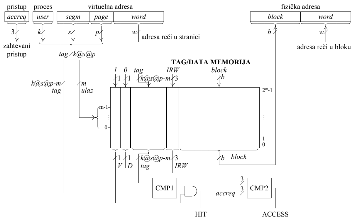
Virtuelna memorija segmentno stranične organizacije i jedinica sa direktnim preslikavanjem
