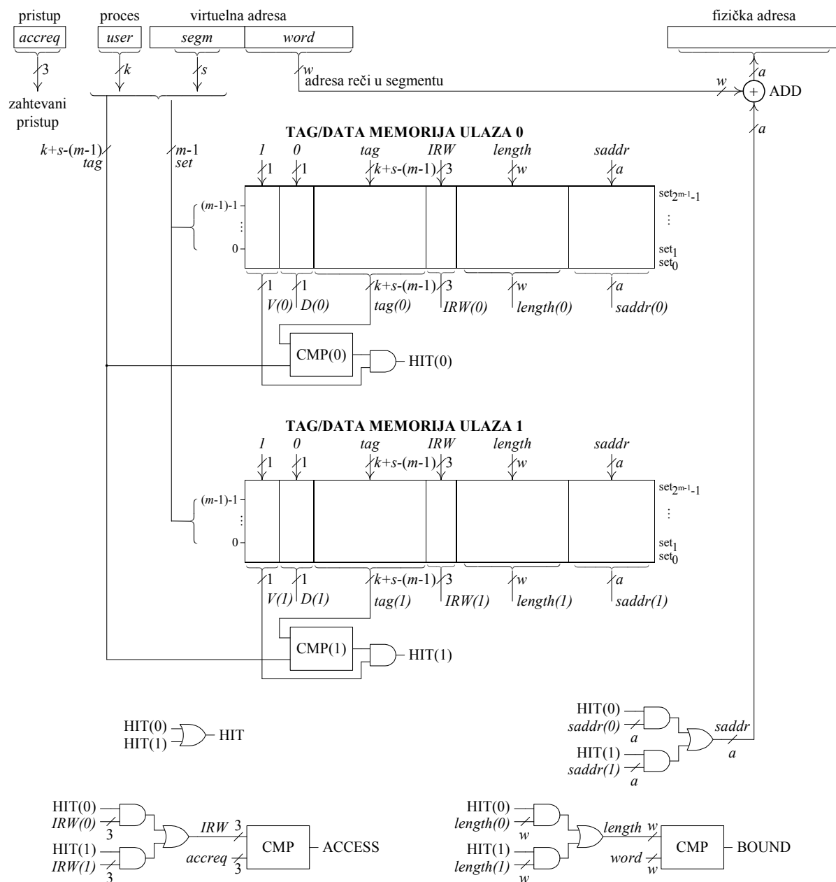
Virtuelna memorija segmentne organizacije i jedinica sa set asocijativnim preslikavanjem
