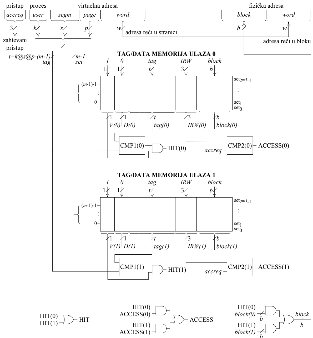
Virtuelna memorija segmentno stranične organizacije i jedinica sa set asocijativnim preslikavanjem
