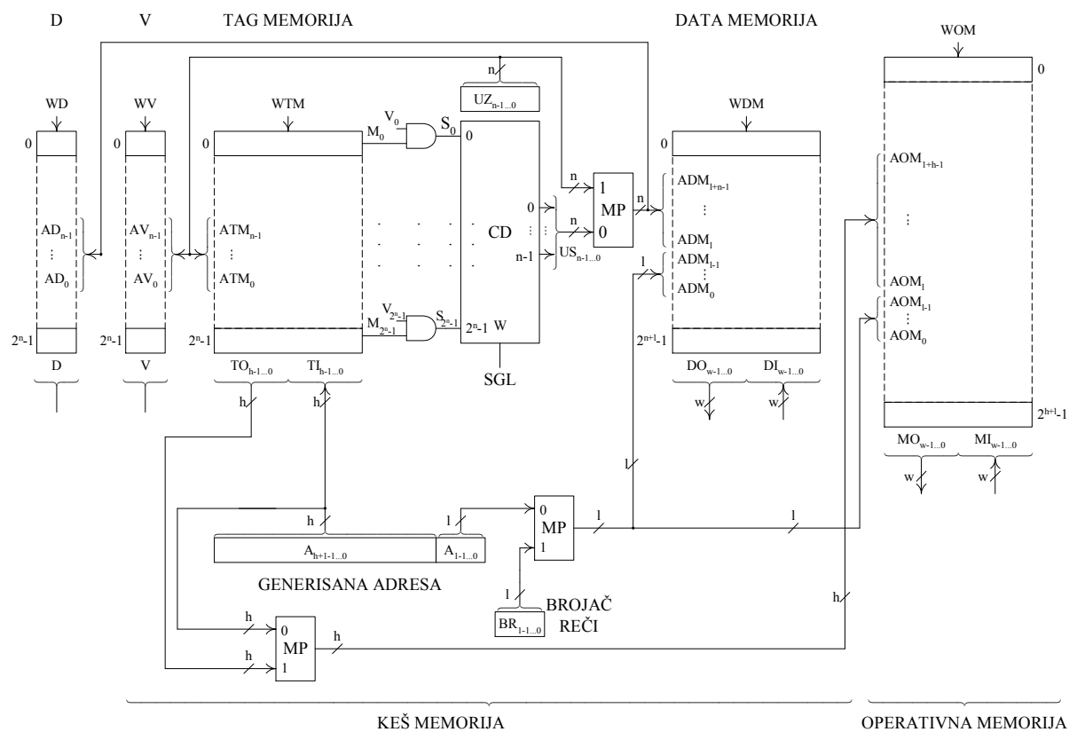
Keš memorija sa asocijativnim preslikavanjem
