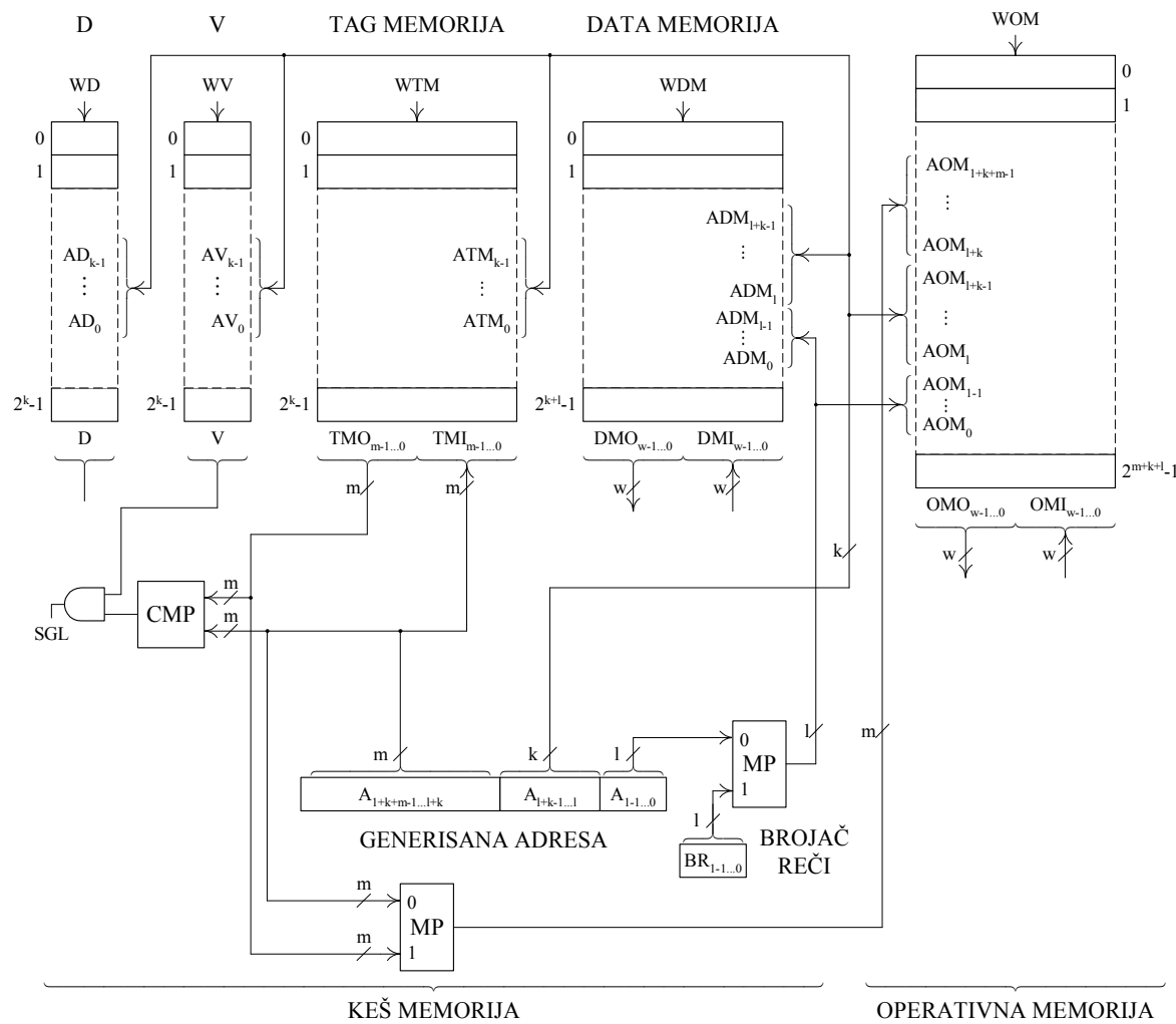
Keš memorija sa direktnim preslikavanjem
