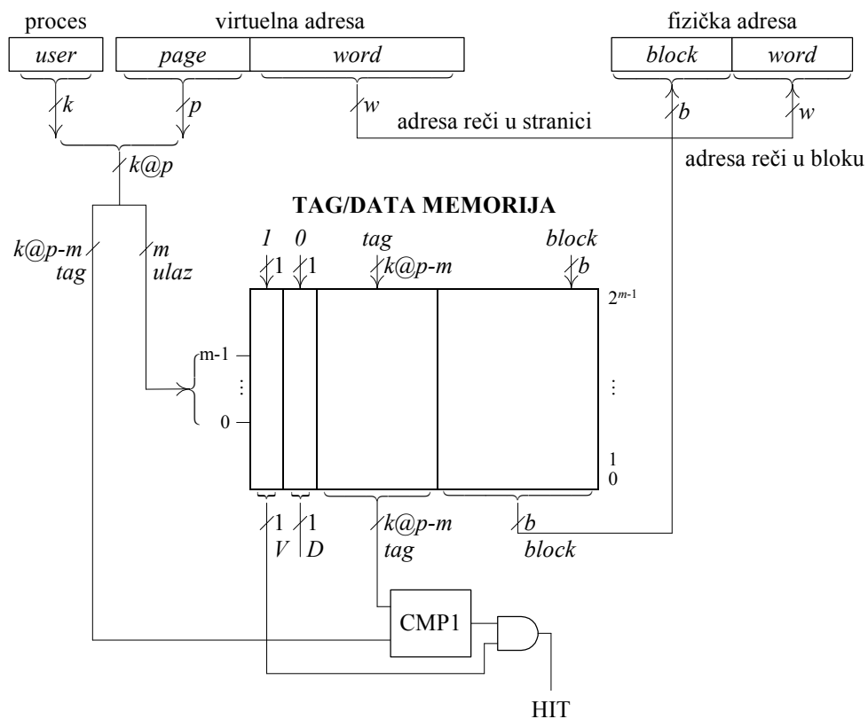
Virtuelna memorija stranične organizacije i jedinica sa direktnim preslikavanjem
