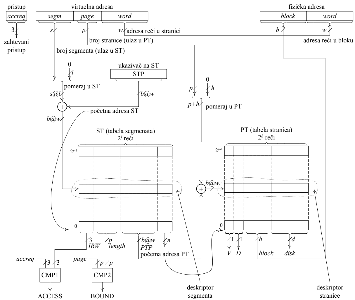
Virtuelna memorija segmentno-stranične organizacije
