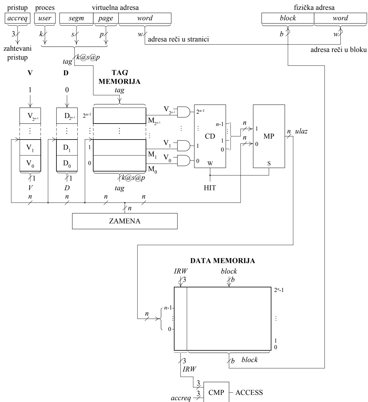
Virtuelna memorija segmentno stranične organizacije i jedinica sa asocijativnim preslikavanjem
