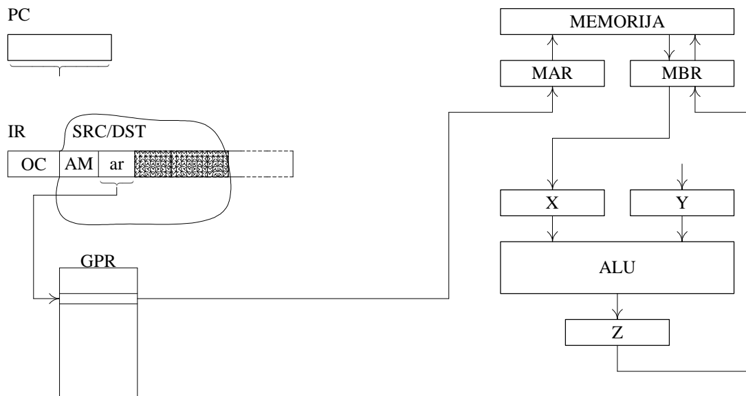
Slika 16 Registarsko indirektno adresiranje
