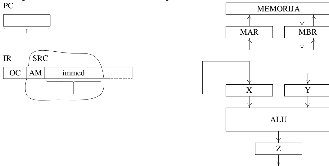
Slika 25 Neposredno adresiranje
