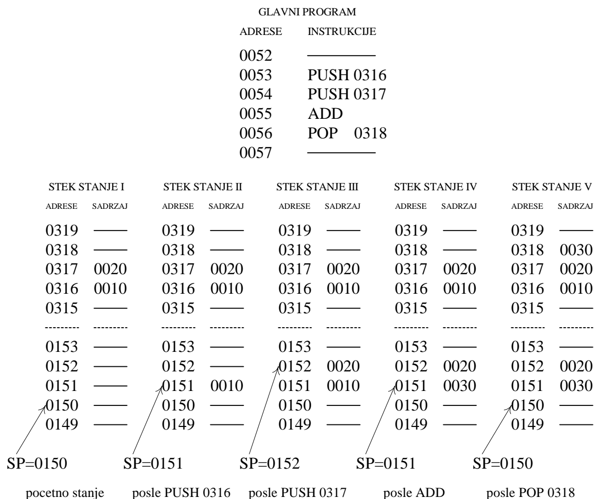
Slika 7 Aritmetički stek
