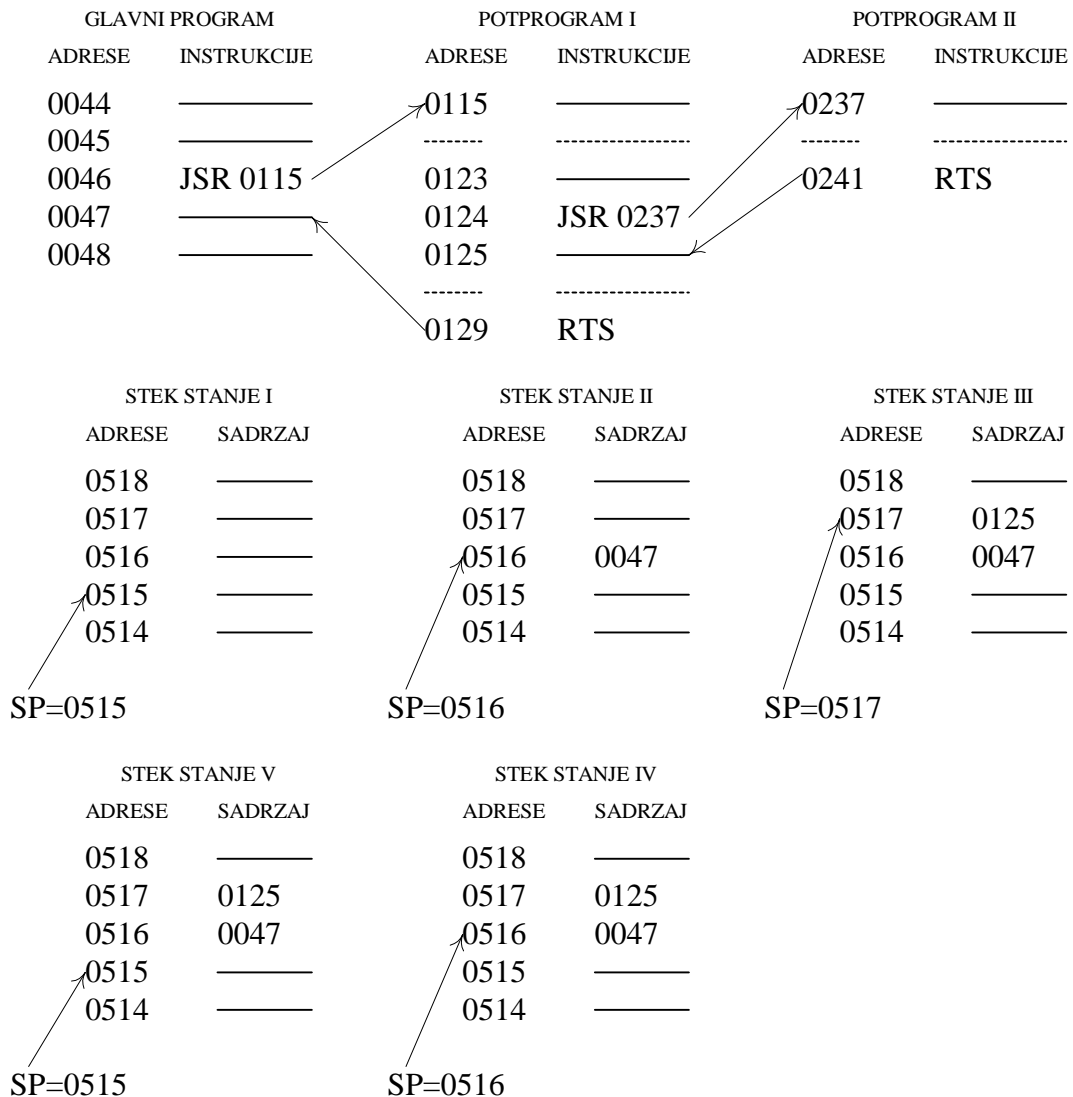
Slika 6 Upravljački stek
